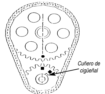
Figura 8 4° Retardado
