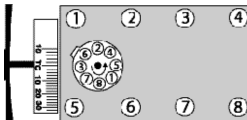
Figura 2 - Ford V8 de 289 a 302 c.i.d. Orden de disparo: 1-5-4-2-6-3-7-8
