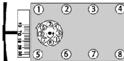
Figure 2 - Ford V8, cylindrée 289-302 Ordre d'allumage : 1-5-4-2-6-3-7-8 Tournez le distributeur dans le sens horaire pour avancer le calage.
